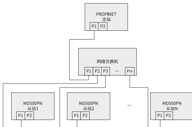
图2-4 星型连接拓扑图
