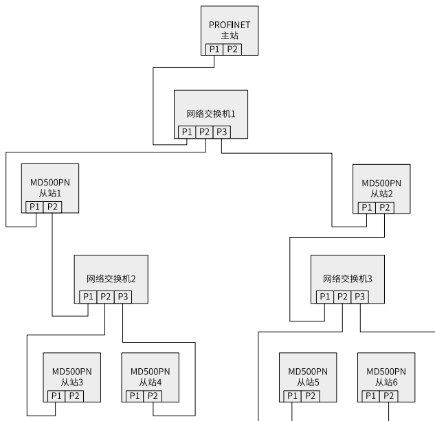
图2-5 树型连接拓扑图
