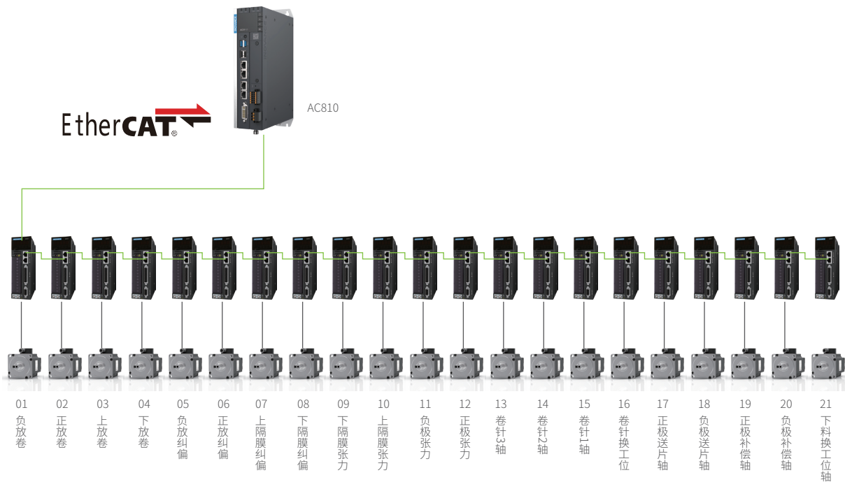
电控系统架构
